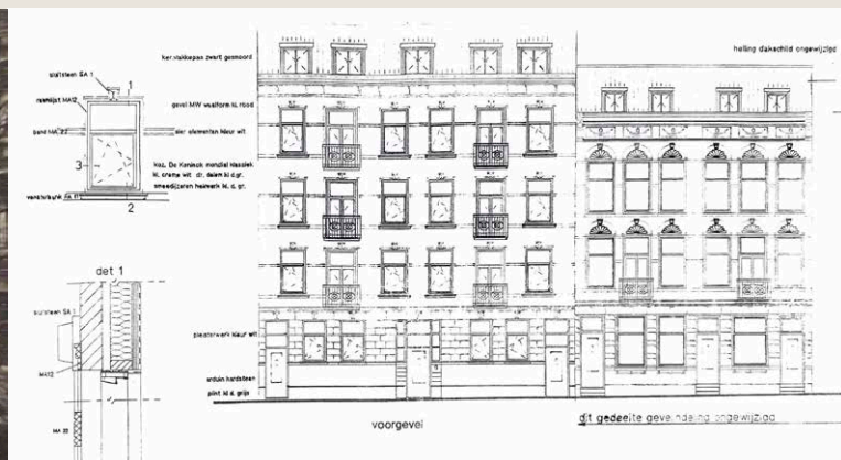
25/10/1999 SAR/Bowoto geveltekening Provenierssingel
